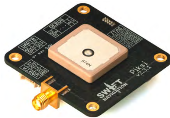
Figura 9. GPS RTK Piksi.
