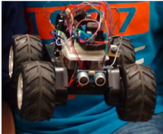
Figura 7. Robot Rover.
